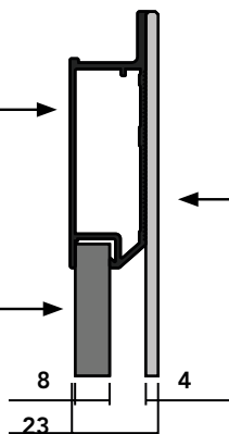
Pannello in vetro/gres/Corian Panneau en verre/grès/Corian Panel in glass/gres/Corian Panel en vidrio/gres/Corian
